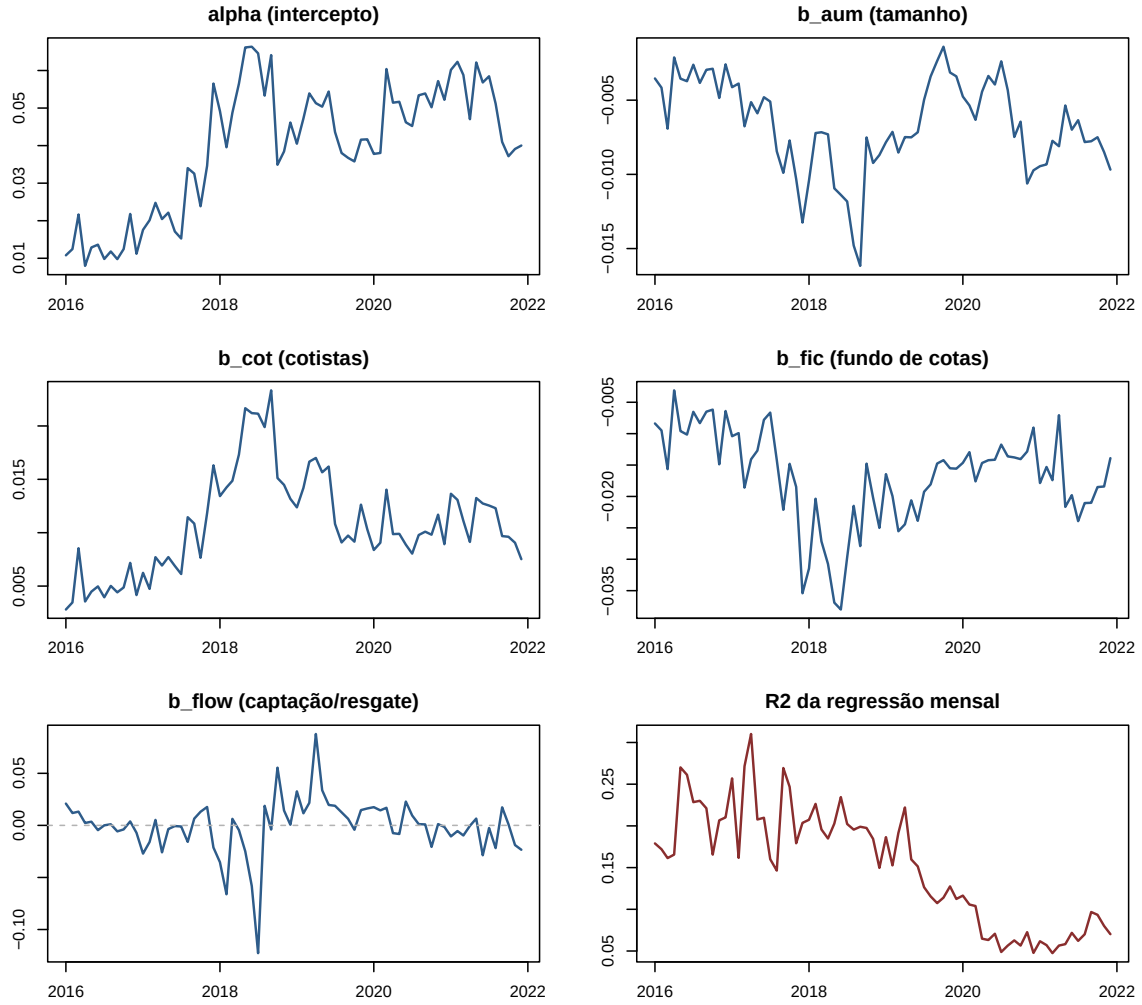
Figura 1: Os cinco componentes de \theta_t ao longo dos 72 meses, e o R^2 de cada regressão mensal. Os coeficientes não são constantes — há uma mudança de patamar visível em torno de 2018 — mas mantêm o mesmo sinal na maior parte do período.
