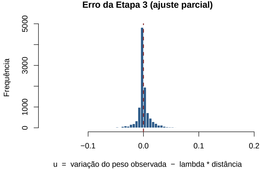
Figura 3: Histograma do erro u da Etapa 3 (10.972 observações). Note o pico estreito perto de zero e as caudas longas — coerente com a curtose alta.
