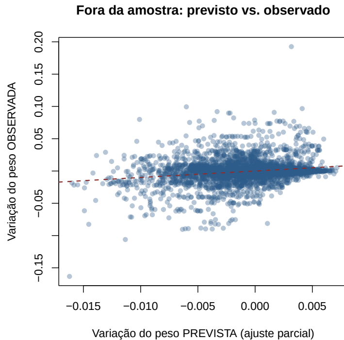
Figura 6: Variação do peso prevista (eixo x) vs. observada (eixo y), fora da amostra. As previsões ficam concentradas perto de zero (o modelo prevê mudanças pequenas), enquanto a variação observada tem bem mais dispersão — coerente com o R^2 baixo da equação (3) (0,038): o modelo capta uma tendência real, mas pequena parte da variação total.
